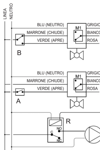
Collegamento del fermo pompa con un servocomando 3 punti ed uno 2 punti
