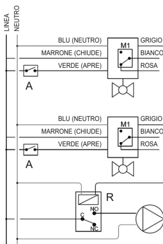
Collegamento del fermo pompa con due servocomandi 2 punti
