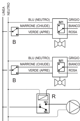
Collegamento del fermo pompa con due servocomandi 3 punti
