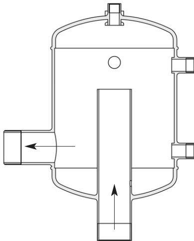
SEZIONE SEPARATORE ATTACCHI A SQUADRA
