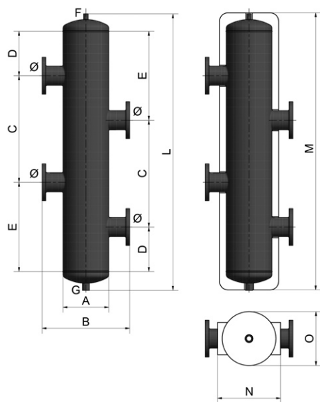
TIPOLOGIA FLANGIA
