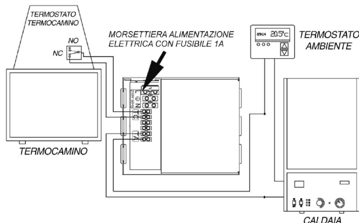
SCHEMA 1 Termocamino dotato di termostato
