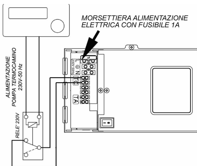
SCHEMA 2 Termocamino dotato di centralina
