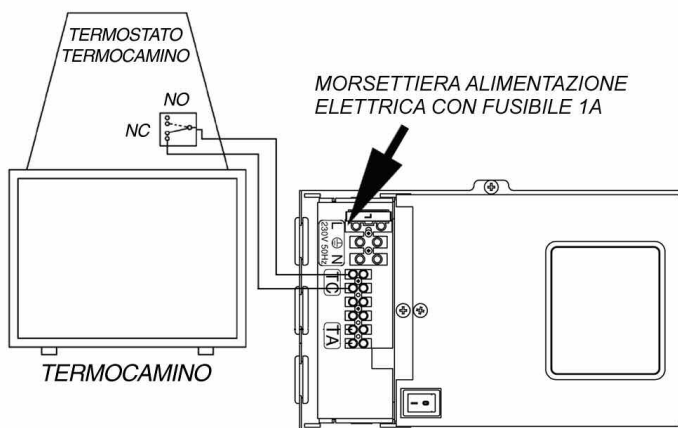
SCHEMA 2 Termocamino dotato di centralina
