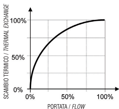
CURVA CARATTERISTICA SCAMBIATORE DI CALORE CHARACTERISTIC CURVE HEAT EXCHANGER
